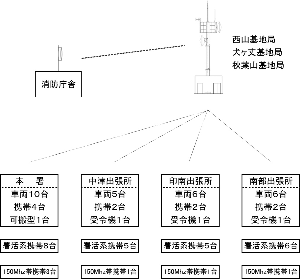
第11表 無線通信構成図
