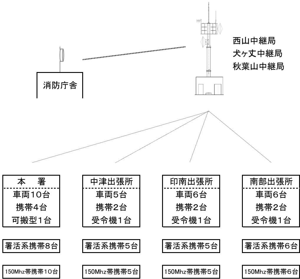
第11表 無線通信構成図
